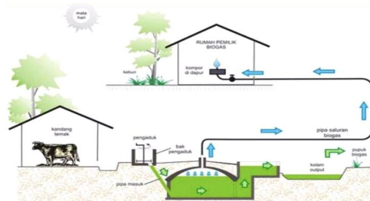
Gambar 26. Ilustrasi pemanfaatan biogas dari industri peternakan sapi
